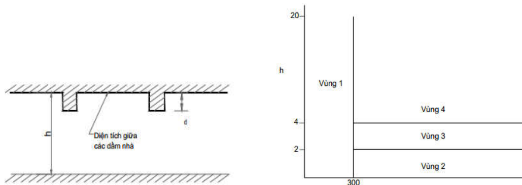
Hình 4 - Yêu cầu thiết kế cho các đầu báo cháy khói kiểu điểm và các hệ thống đầu báo cháy khói kiểu hút trong các cấu trúc nhà có dầm
