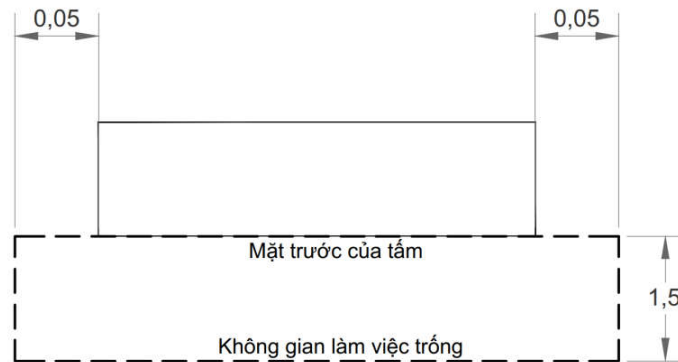
Hình 10 - Khoảng hở nhỏ nhất đến kết cấu bao che khu vực bảo vệ
