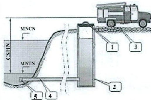
Hình H.2. Quy cách đường ống dẫn và hố thu nước cho xe chữa cháy lấy nước. CHÚ DẪN
