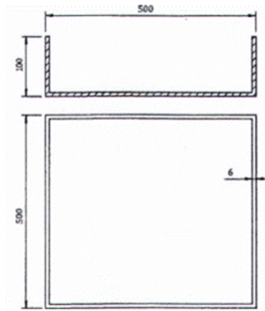
Hình C.7 - Kích thước của khay để thử đốt cháy củi gỗ và khay heptan
