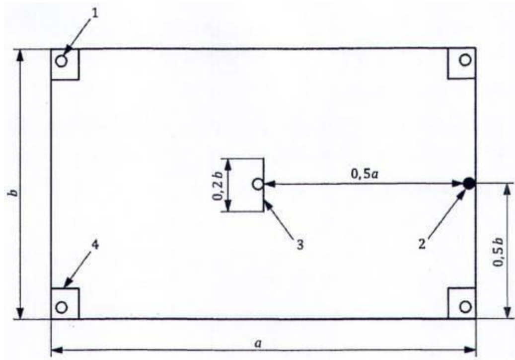
Hình C.1 - Ví dụ sơ đồ để thử chiều cao nhỏ nhất/ diện tích quét lớn nhất của đầu phun loại 360^\circ
