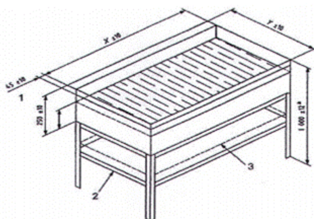
Hình 4- Các kích thước chung đối với thiết bị thử đám cháy loại F - Thiết bị thử kiểu A chỉ dùng cho loại đám cháy 5F
