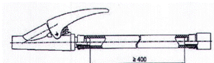
Hình 8 - Chiều dài nhỏ nhất của ống mềm
