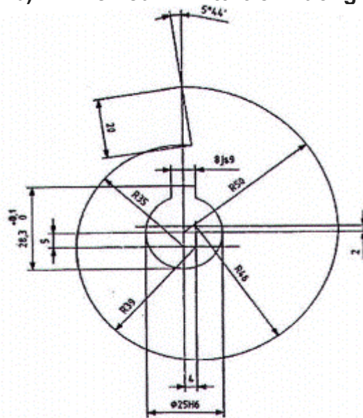
c) Cam - chi tiết số 9 của Hình 1a
