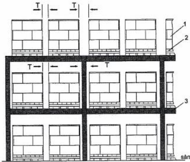
Hình A.5 - Minh họa phương án bố trí khe khối ngang
