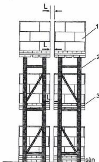
Hình A.3 - Minh họa phương án bố trí các kệ hàng nhiều dãy
