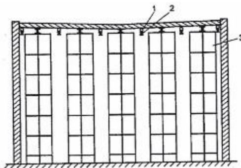
Hình 1 - Minh họa phương án bố trí các đầu phun phía trên mái
