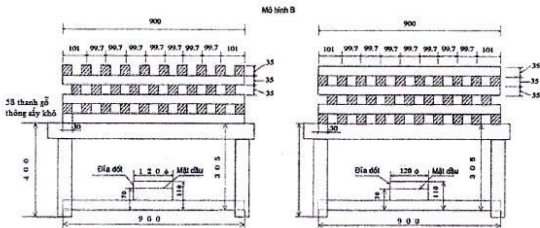
Hình 1 - Mô hình A và B
