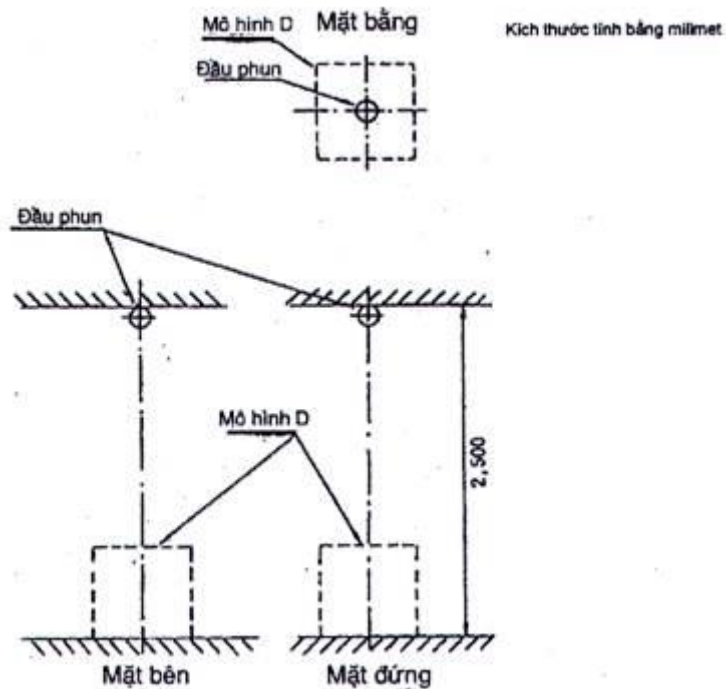
Hình 5 - Bố trí thử nghiệm 2, loại 2
