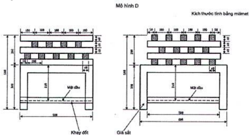
Hình 4 - Mô hình D
